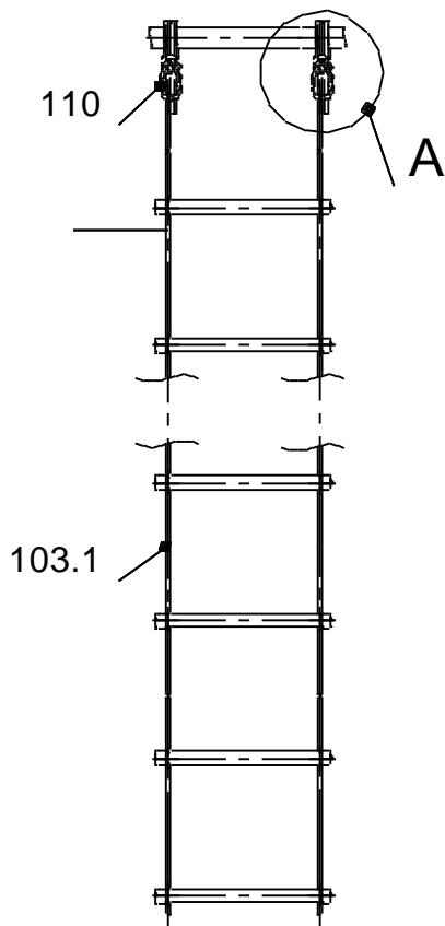
Рис.1. Общий вид лестницы веревочной
